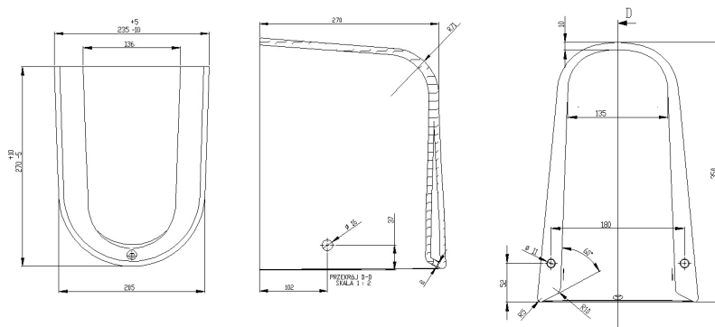
Rysunek techniczny
