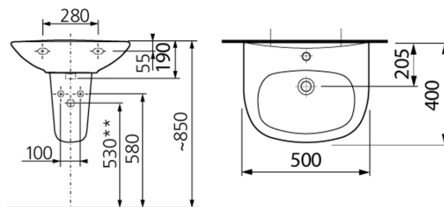
Rysunek techniczny
