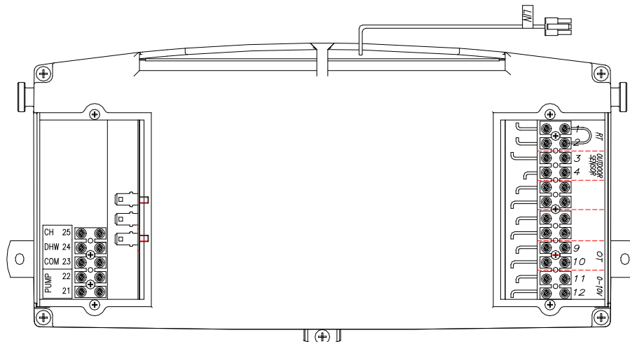
Rys.3.9.1.a Zaciski elektryczne sterownika kotłów dwufunkcyjnych
