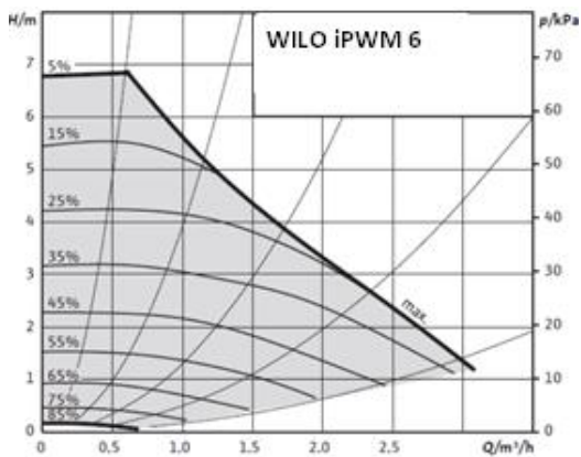
Charakterystyka pompy dla kotłów RED BY TERMET II 20 i 25kW;
