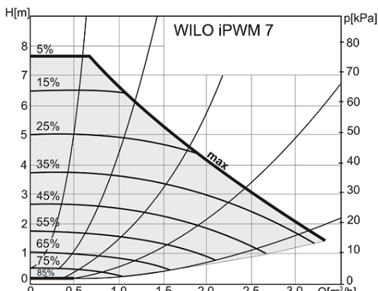
Charakterystyka pompy dla kotłów RED BY TERMET II 35kW.
