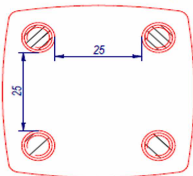
Przekrój A-A
