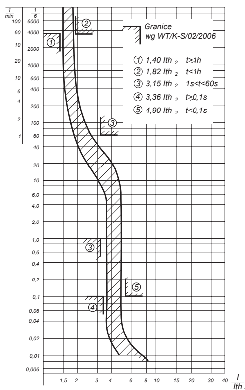
Charakterystyka L, I_{th2}=16-25 A
