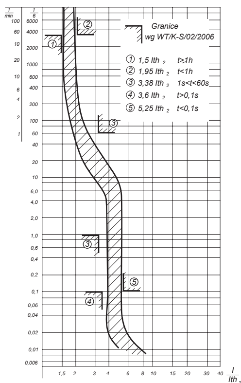
Charakterystyka L, I_{th2}=6-10 A
