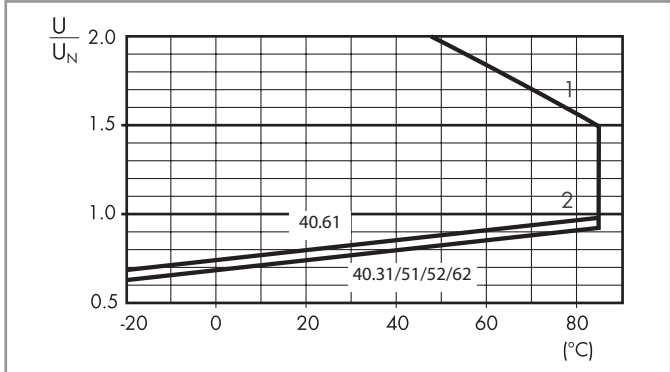
R 40 - DC Dopuszczalny zakres napięcia pracy cewki w zależności od temperatury otoczenia - Wykonanie czułe, typy 40.31/51/52/61/62
