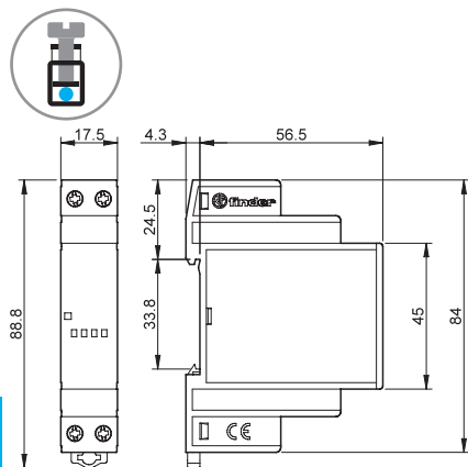
Typ 77.01 Zaciski śrubowe
