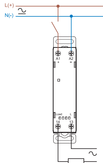
Podłączenie jednofazowe (77.11/77.21)
