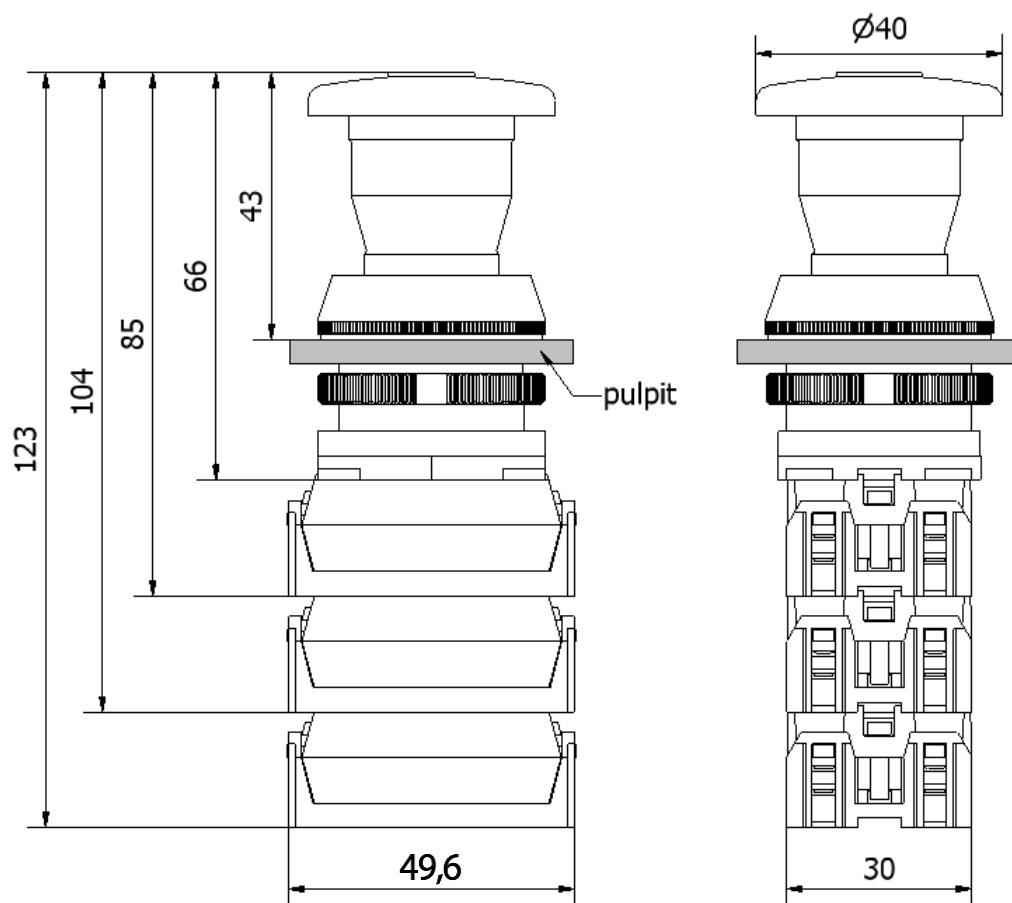
NEF30-UDR
