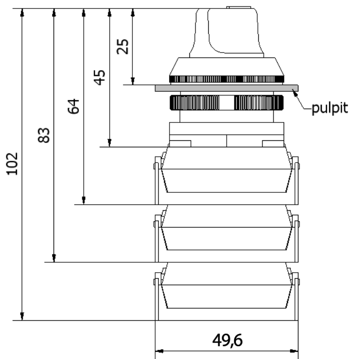
NEF30-TP
