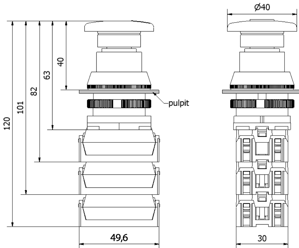
NEF30-DR
