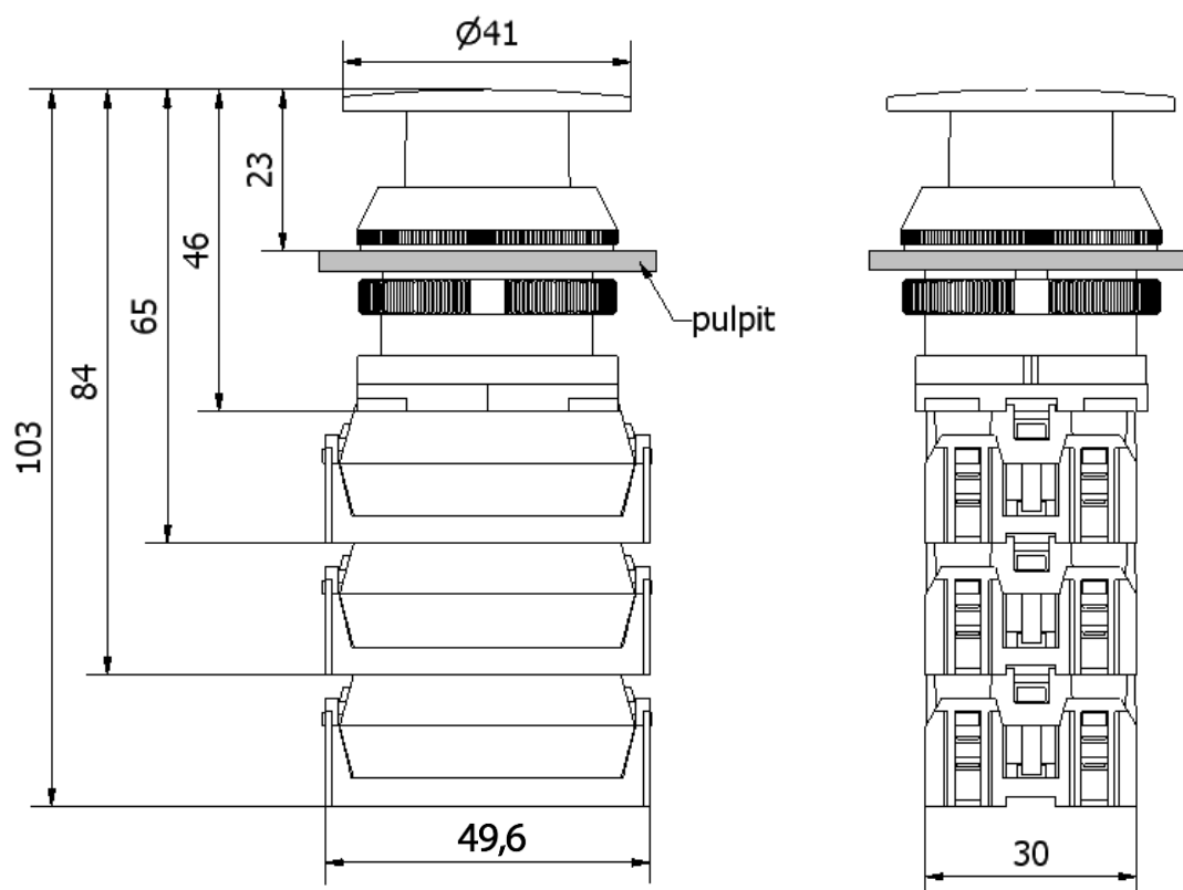
NEF30-D
