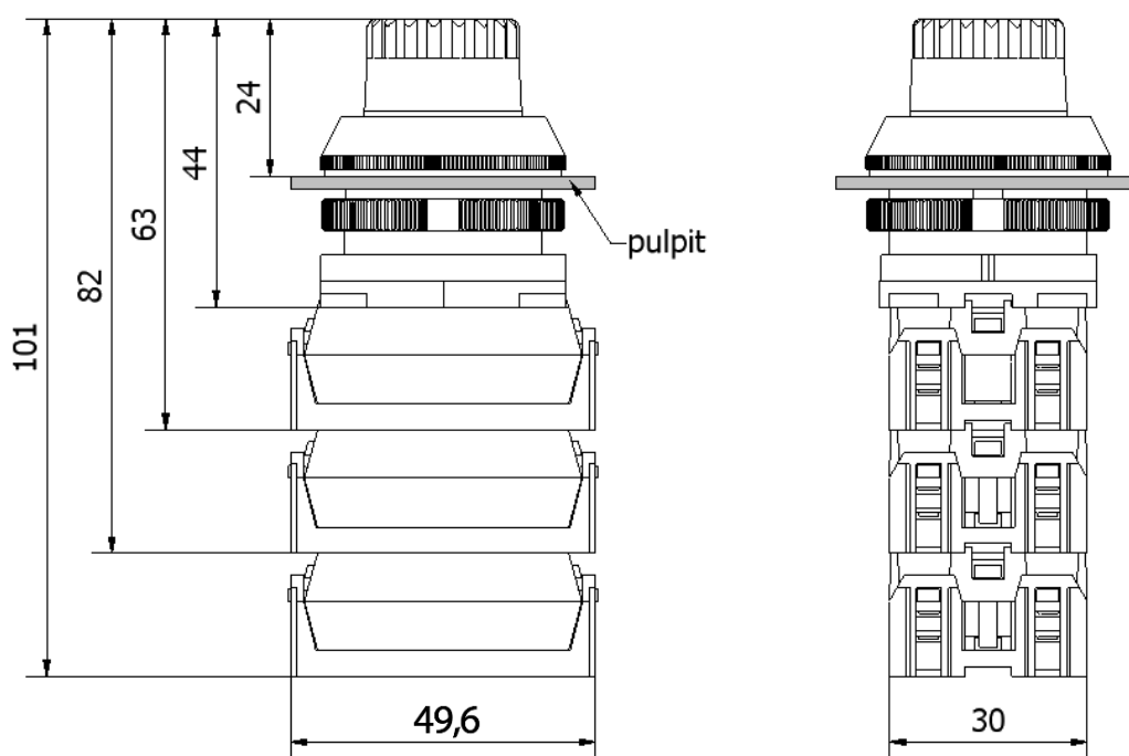
NEF30-WR
