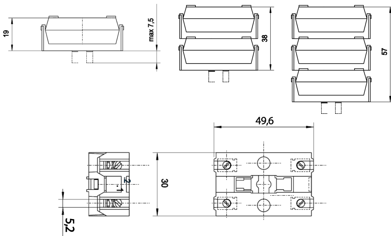
EF30
