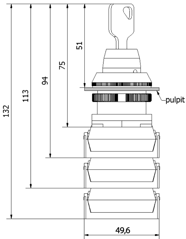
NEF30-B
