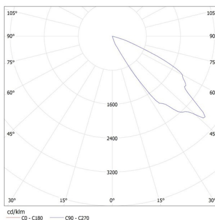
KANLUX S.A. (kat 32495) MEFIS LED W-NW / LDC (Polar)
