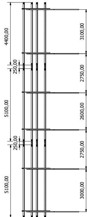
28 paneli / 28 modules
