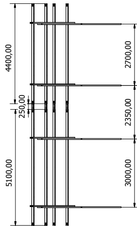
18 paneli / 18 modules
