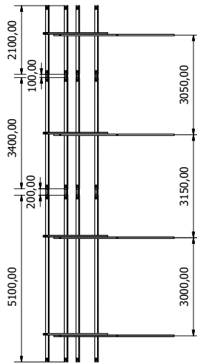
20 paneli / 20 modules
