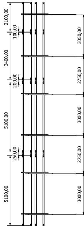
30 paneli / 30 modules
