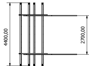
8 paneli / 8 modules
