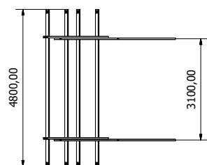
8 paneli / 8 modules
