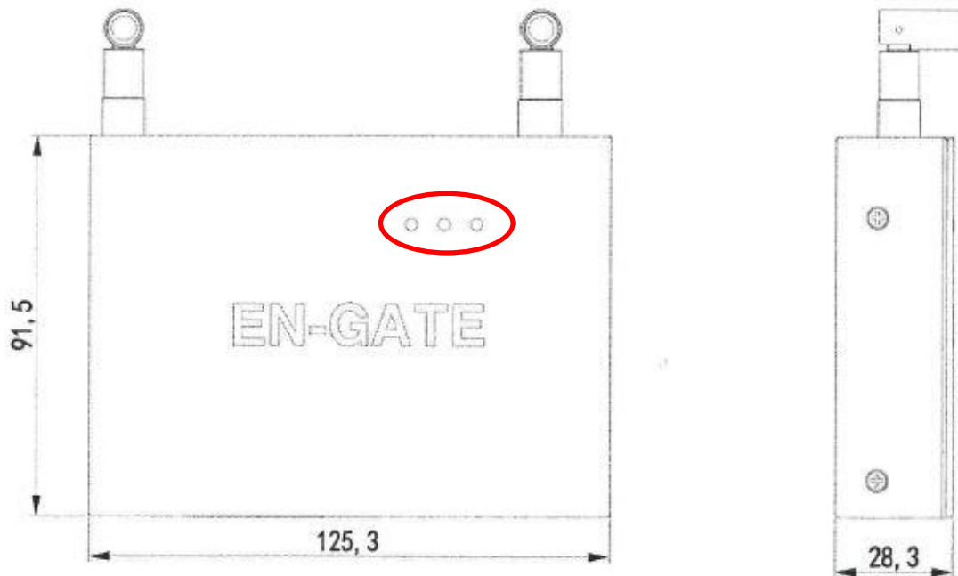
Rysunek 39 - Wymiary urządzenia
